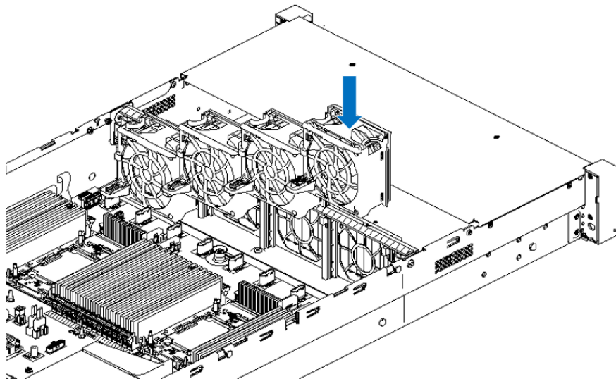
图 3-15 风扇安装示意图
