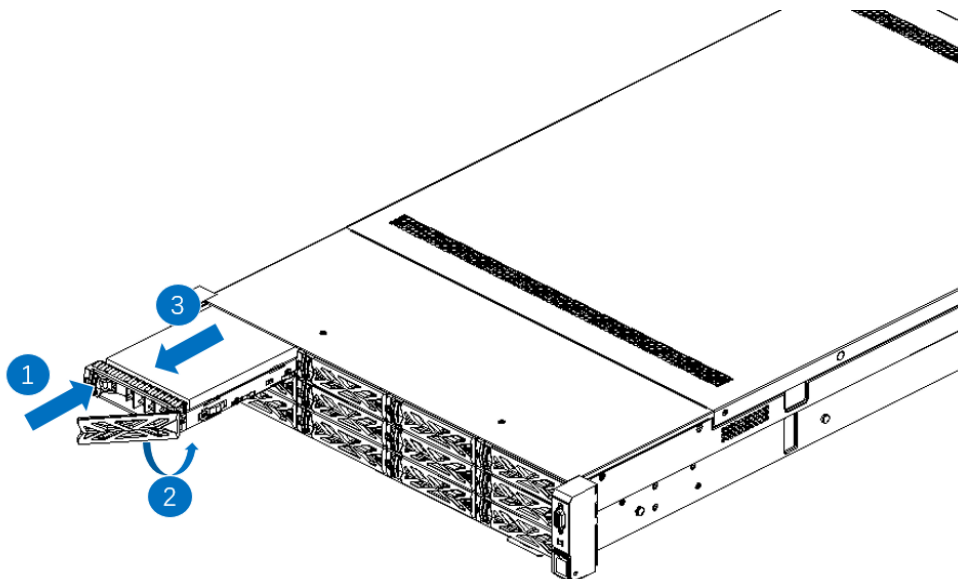
图 3-9 硬盘拆卸示意图
