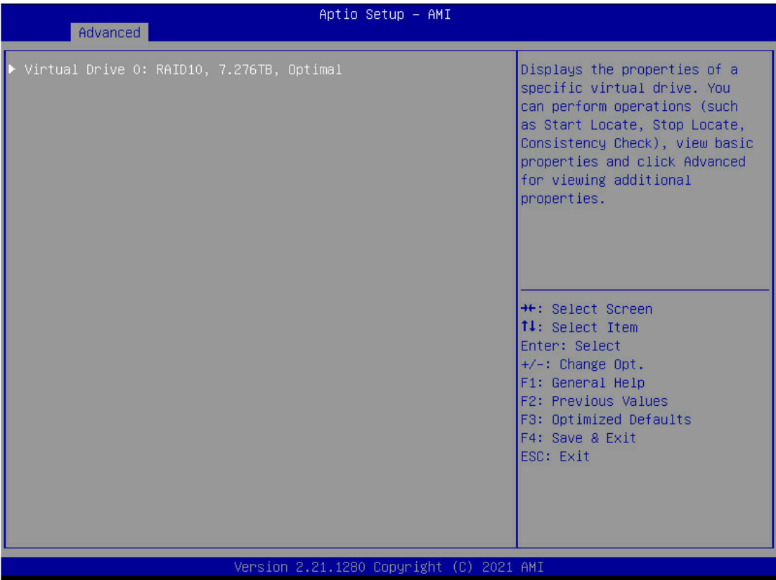
图 7-33 查看 RAID 信息
