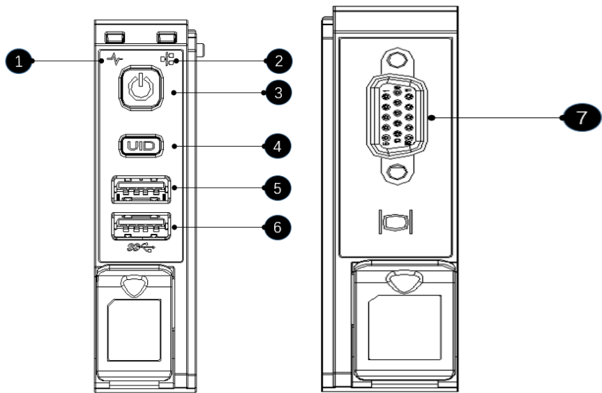
图 2-2 前面板指示灯和接口位置
