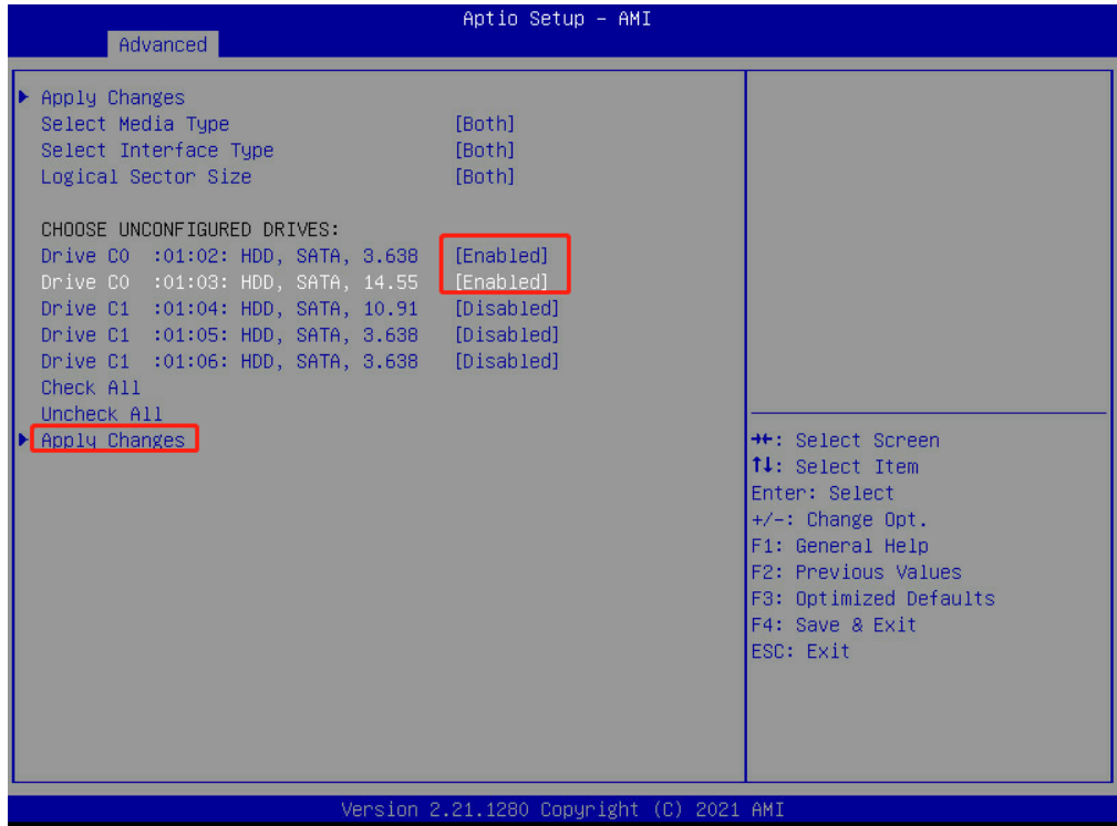
图 7-26 选择要组建 Span1 的硬盘
