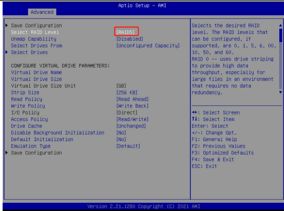
图 7-20 选择 RAID 级别界面，选择 RAID5
