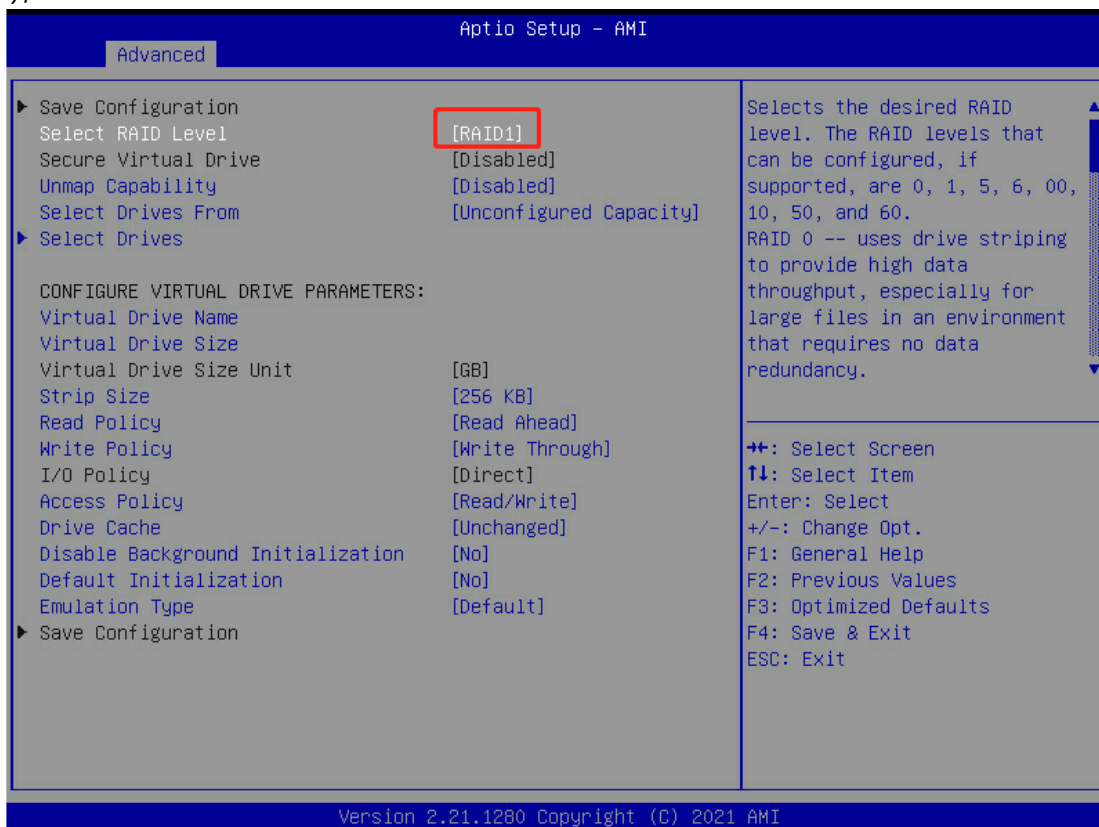
图 7-12 选择 RAID 级别界面
