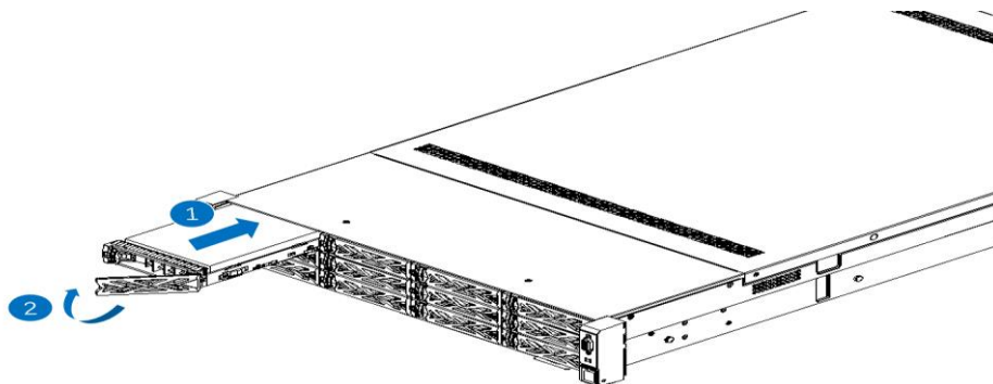
图 3-8 硬盘安装示意图
