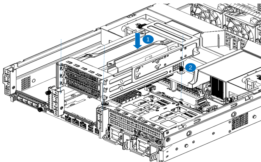
图 3-14 扩展卡模组安装示意图
