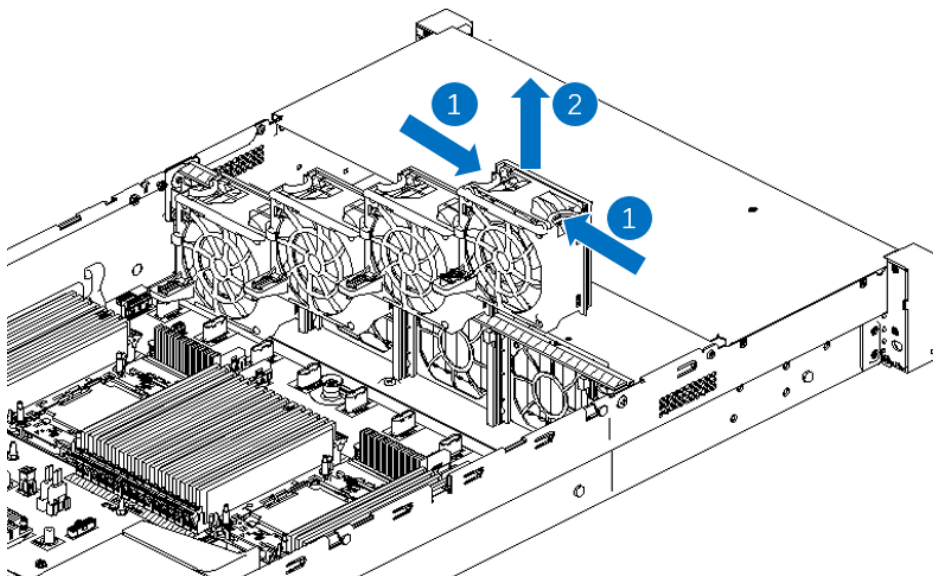
图 3-16 扇拔出示意图
