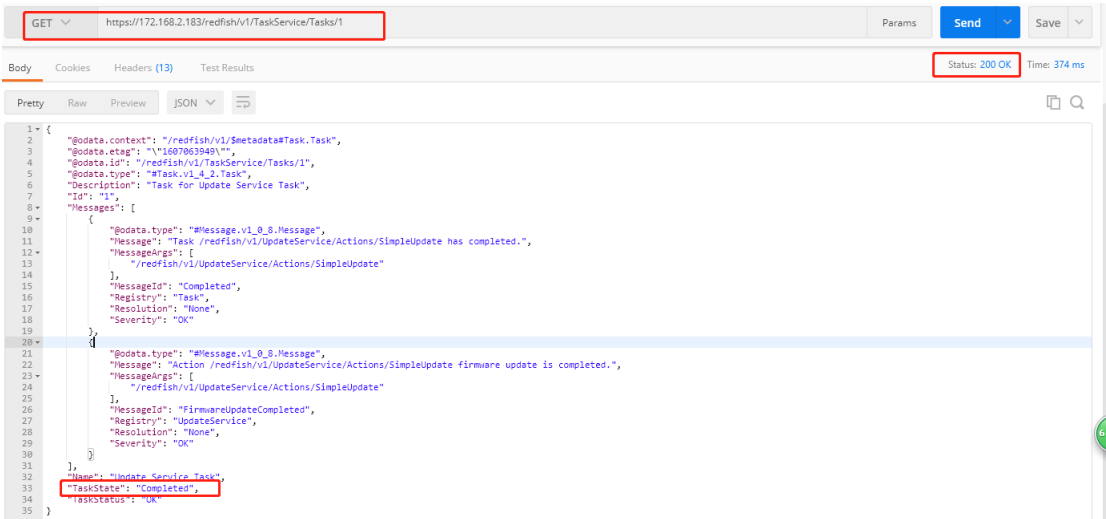
图 8-11 升级任务状态
