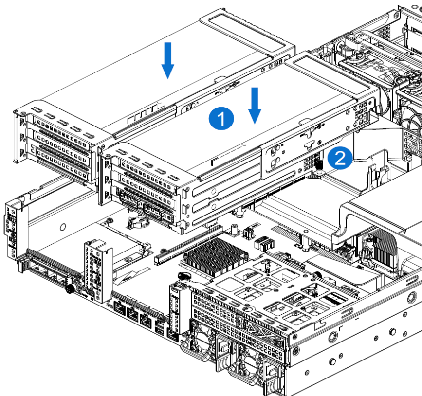
图 3-18 双 GPU 模组安装示意图
