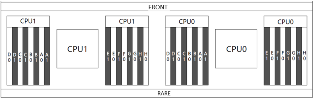
图 2-9 内存插槽位置图
