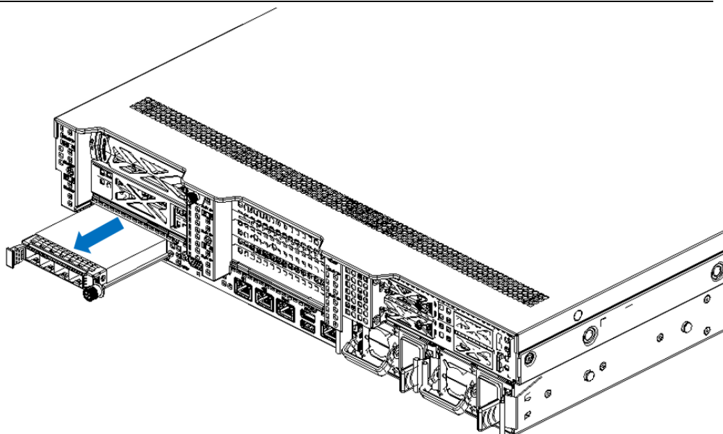
图 3-19 OCP 卡拔出示意图
