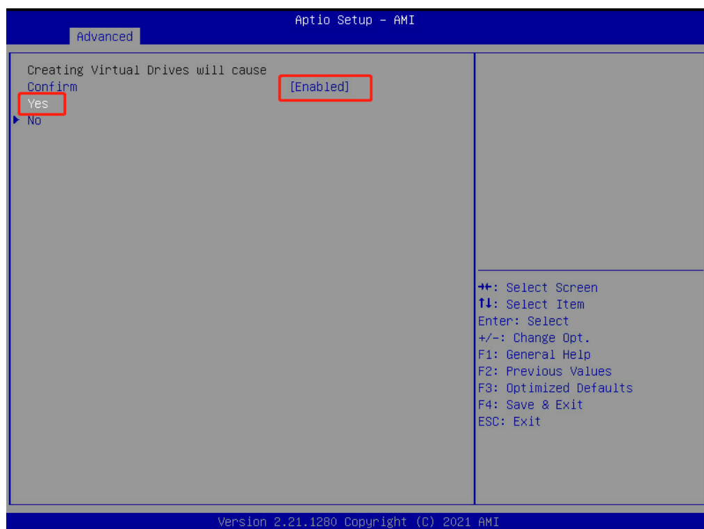
图 7-30 confirm 选择 Enabled 后点击 Yes
