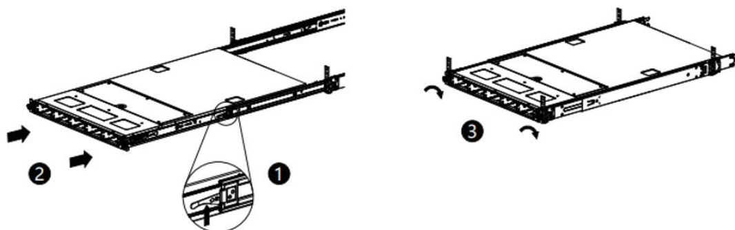
图 3-20 机箱导轨内轨安装
