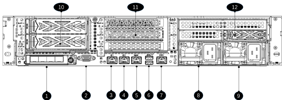
图 2-2 后面板外观 1
