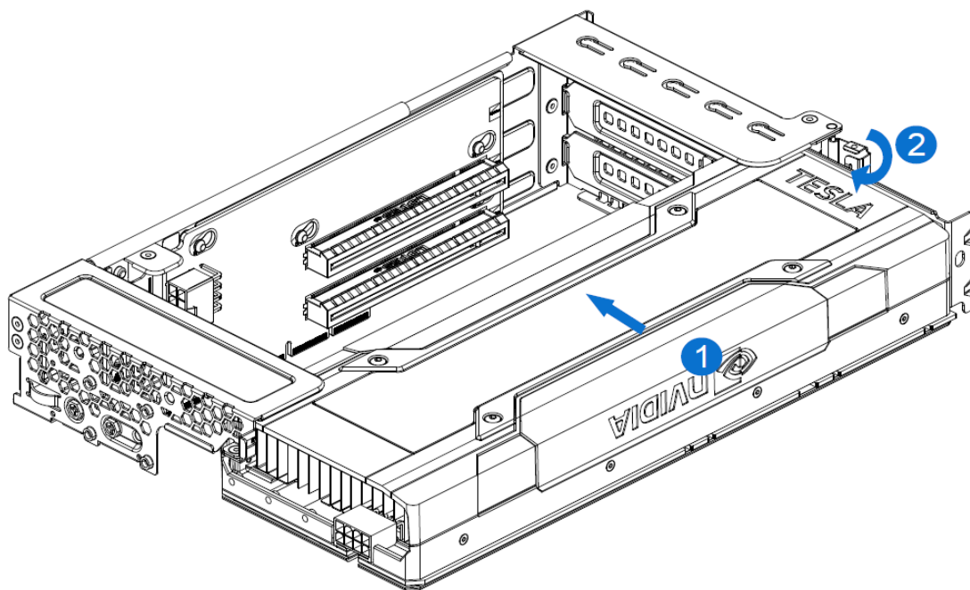
图 3-17 GPU 安装示意图
