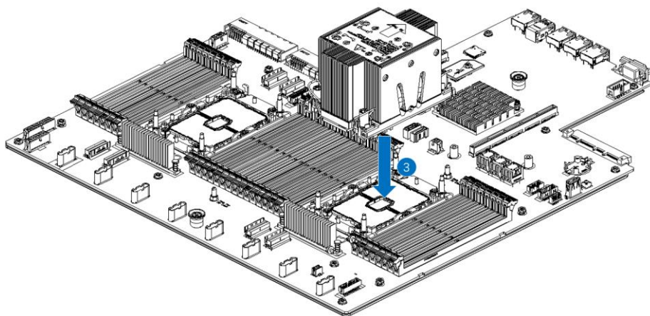
图 3-6 CPU 安装示意图
