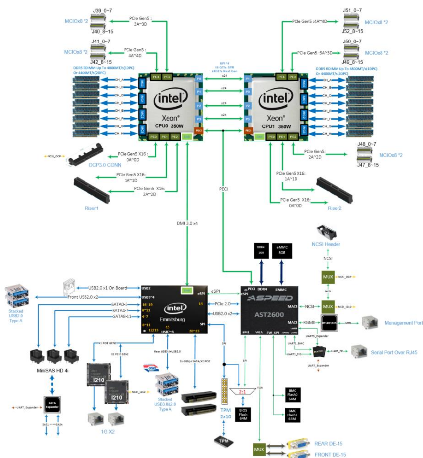
图 2-7 主板架构示意图
