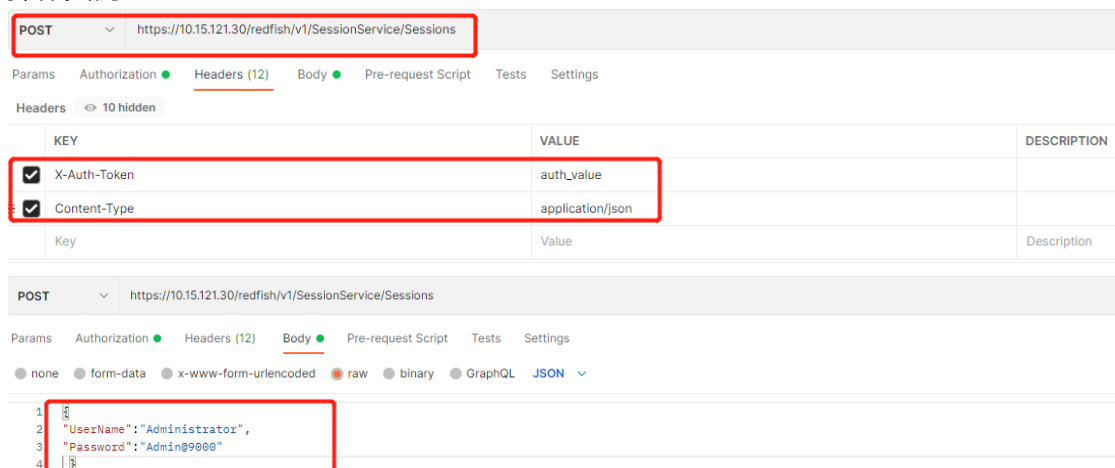
图 5-30 Redfish 升级 BIOS 固件
