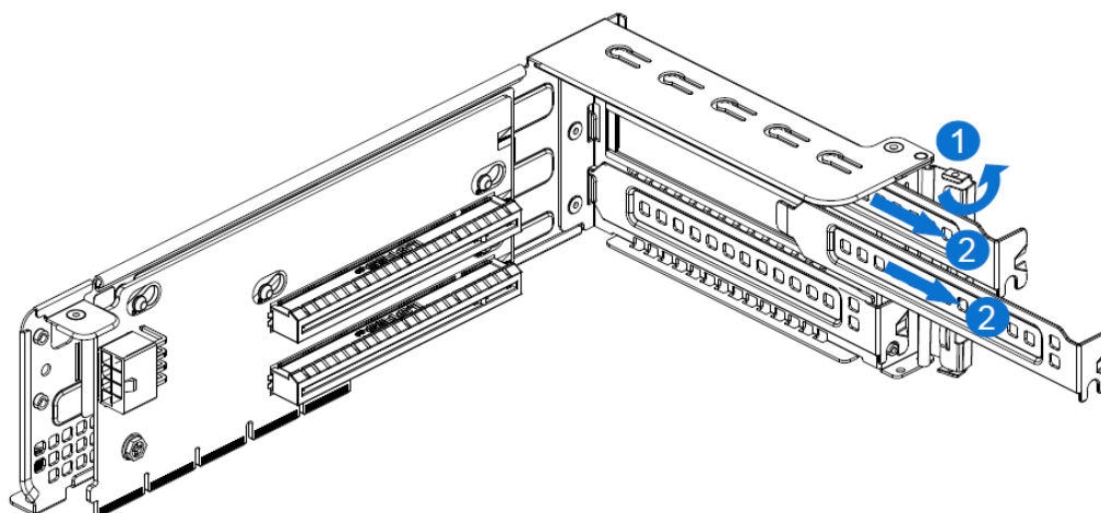
图 3-15 扩展卡支架挡片拆卸示意图
