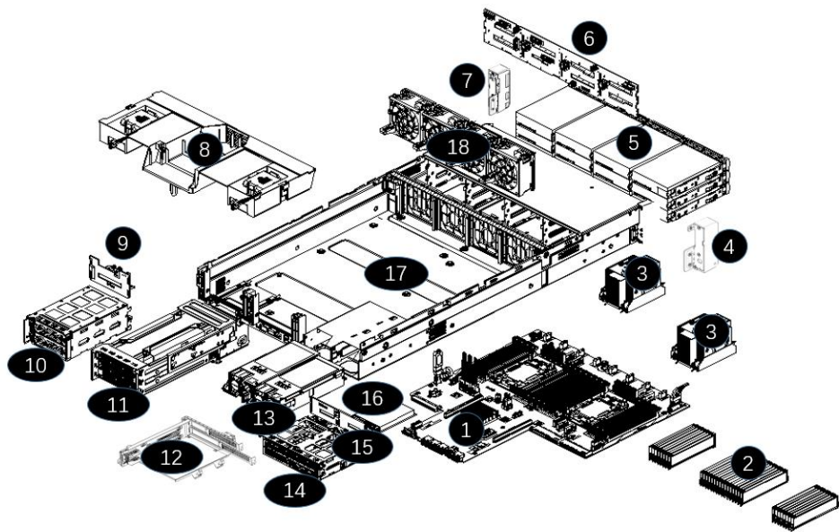
图 2-10 产品布局
