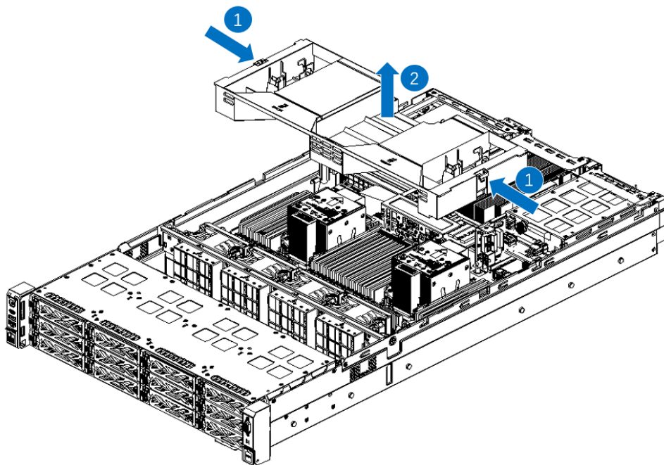
图 3-5 风罩拆卸示意图
