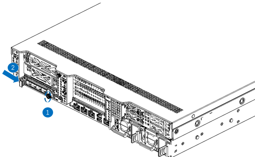
图 3-18 OCP 卡解锁示意图
