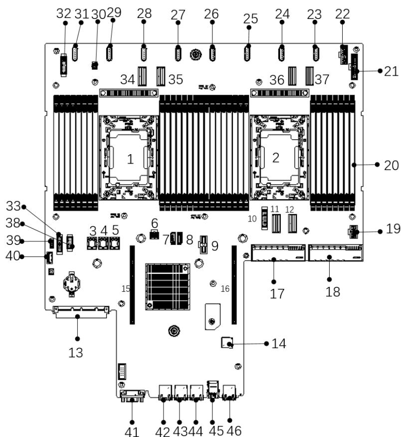
图 2-8 主板接口示意图
