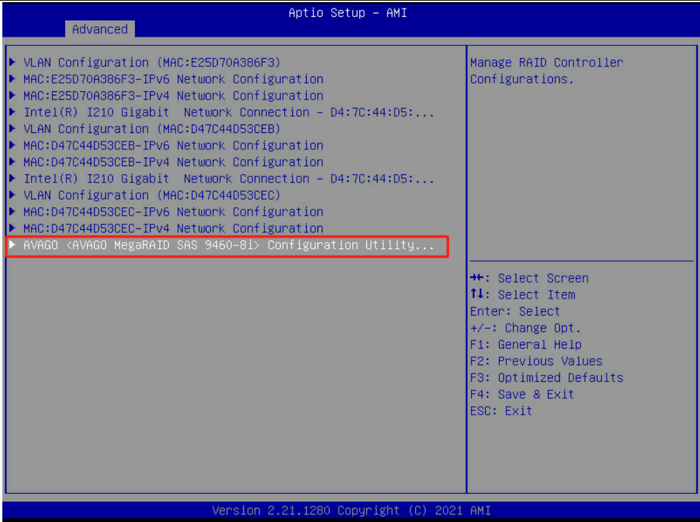
图7-2 Dynamic UEFI Oprom下对应的RAID卡信息
