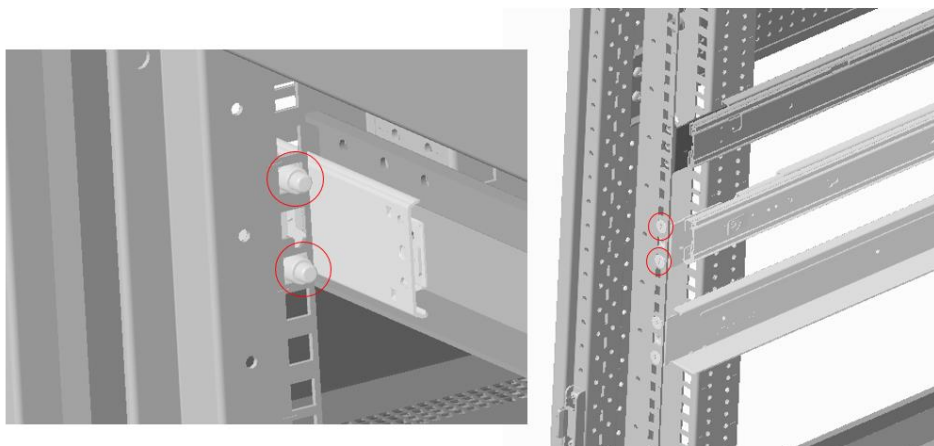
图 3-21 机架导轨外轨安装
