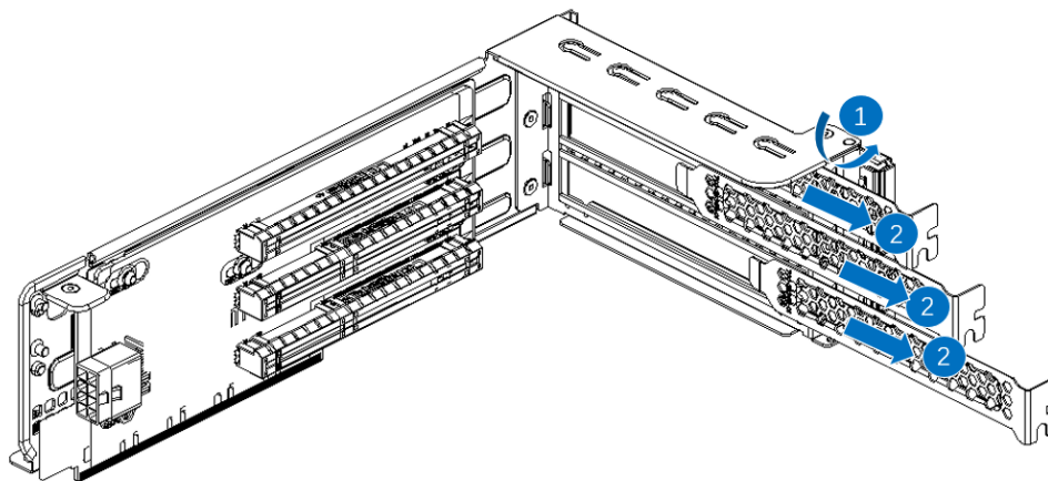
图 3-11 扩展卡支架挡片拆卸示意图
