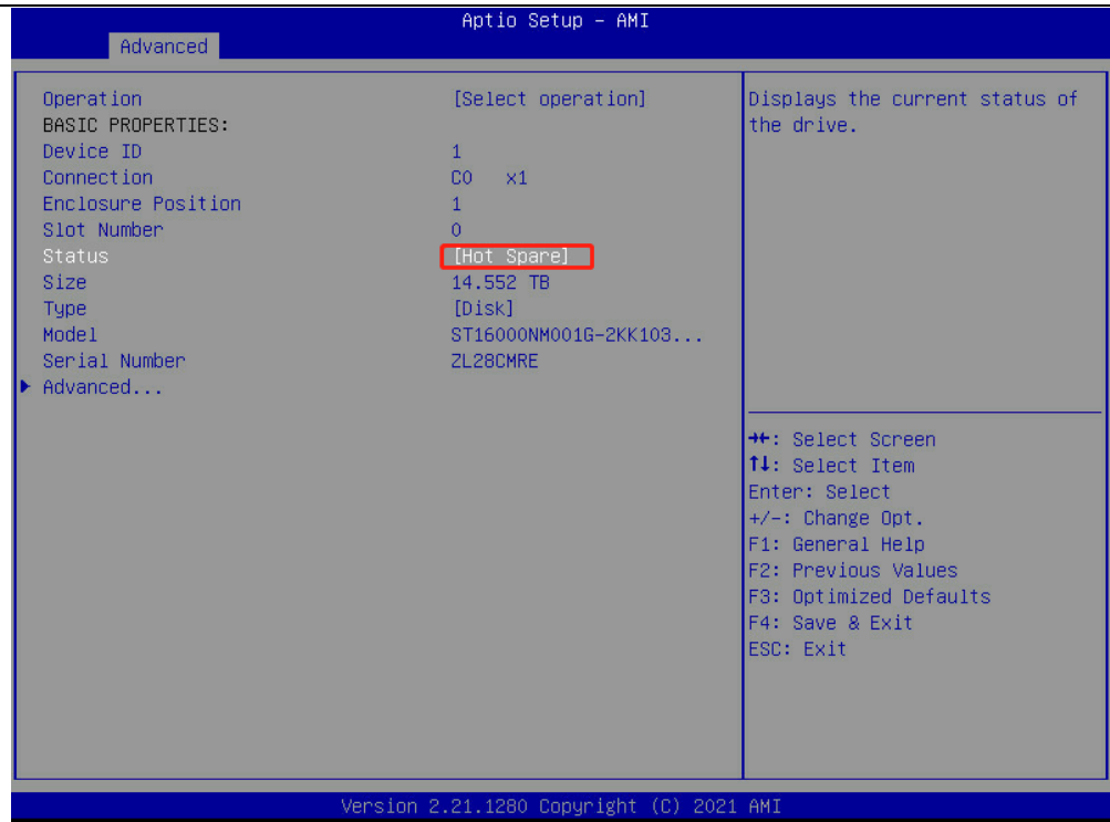
图 7-41 查看硬盘状态
