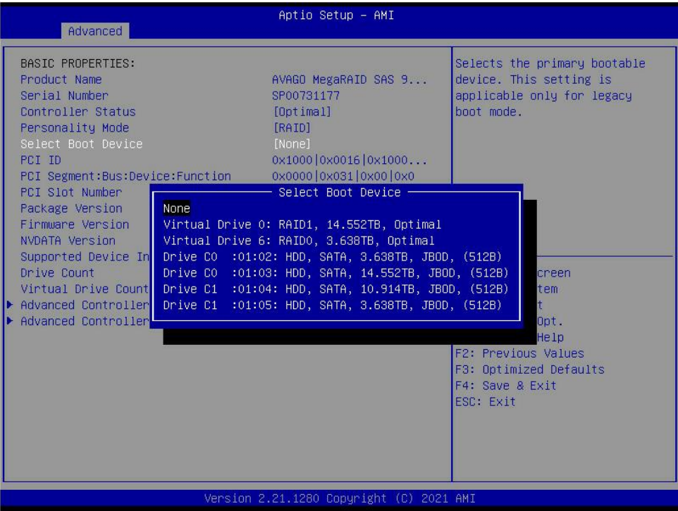
图 7-54 Select Boot Device
