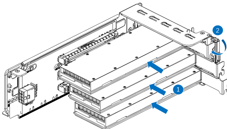
图 3-12 扩展卡安装示意图
