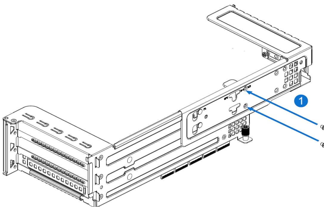
图 3-16 GPU 支架安装示意图
