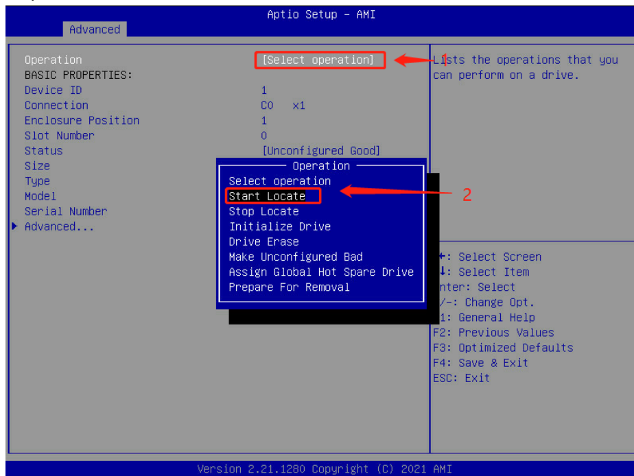
图 7-57 选择 Start Locate
