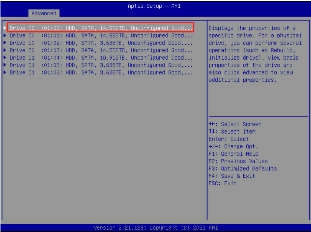
图 7-37 选择一个硬盘按 Enter 进行热备设置
