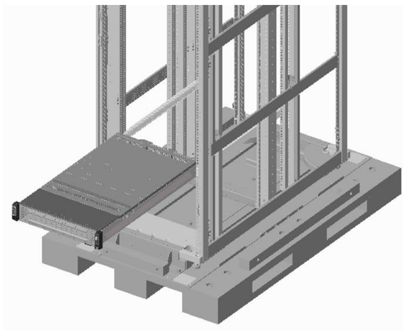
图 3-22 机箱上架安装
