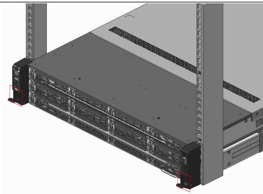
图 3-23 机箱固定
