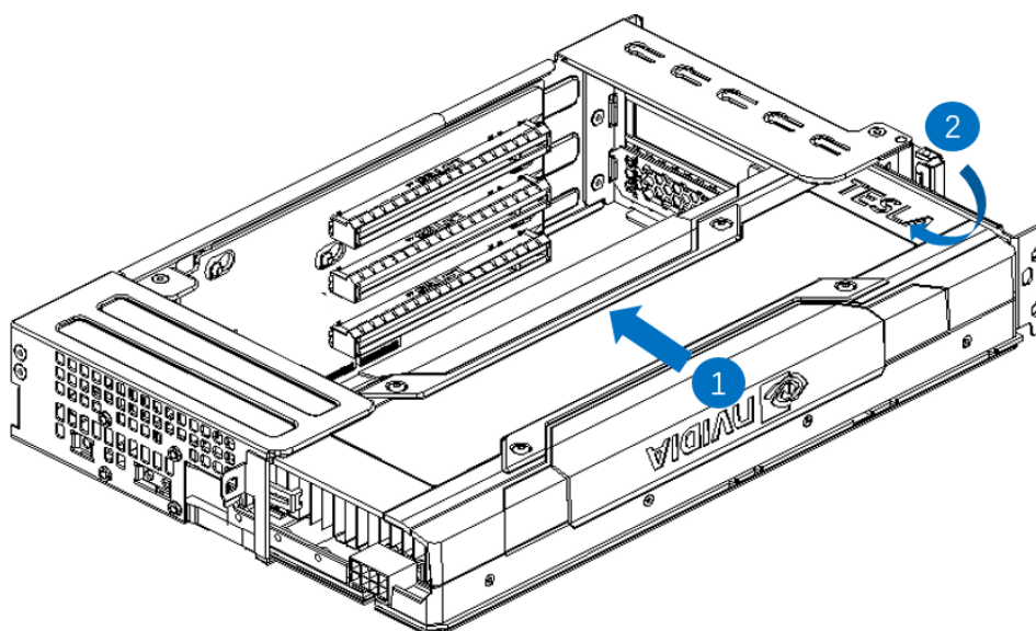
图 3-13 GPU 卡安装示意图
