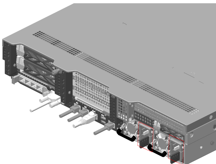
图 3-3 机箱外部接线图
