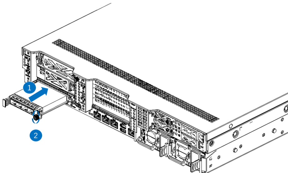
图 3-17 OCP 卡安装示意图
